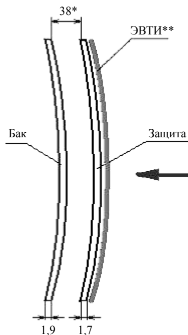
Рис. 5. Фрагмент бака с установленной противометеорной защитой
