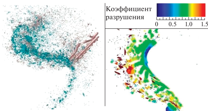
Рис. 3. Облако фрагментов и степень поврежденности ударника при ударе под углом 45^\circ с увеличением шага сетки в \sqrt{2} раз (схема на рис. 1б). Время t = 5 мкс.
