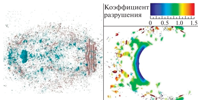
Рис. 2. Облако фрагментов и степень поврежденности ударника для удара по нормали (схема на рис. 1а). Время t = 5 мкс.
